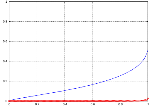
(d) Set 4: f_2(x) (solid) and f_3(x) (circles)
