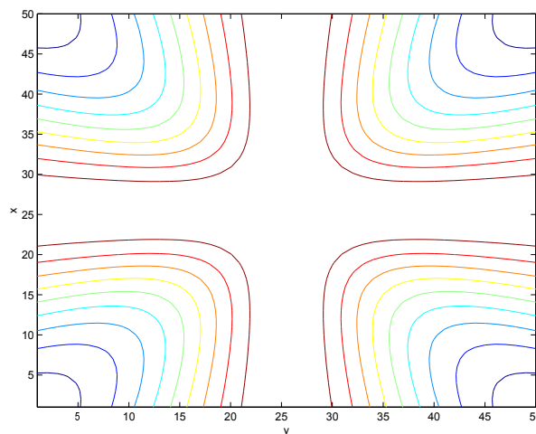
Figura 1.2.: Curvas de nivel de \text{sen}\left(\frac{xy}{x^2+y^2+1}\right)
