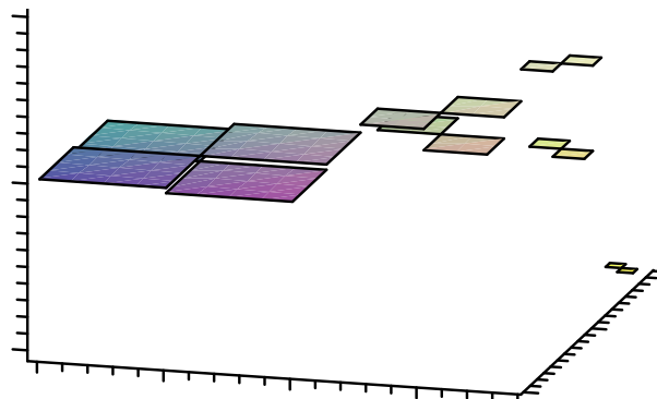
Figura 3.6.: La función del ejemplo 3.4.
