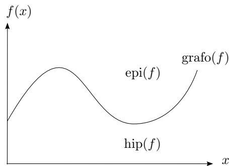
Figura 2.1.: Epígrafo, hipografo y grafo de una función
